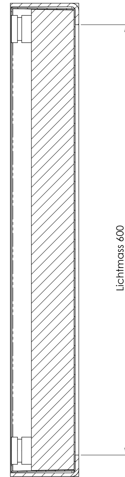
SCHNITT B-B MABSTAB 1 : 3
